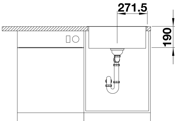
Вид спереди
