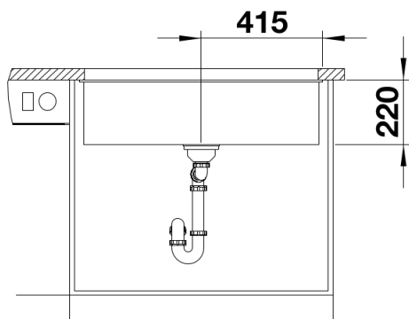
Вид спереди
